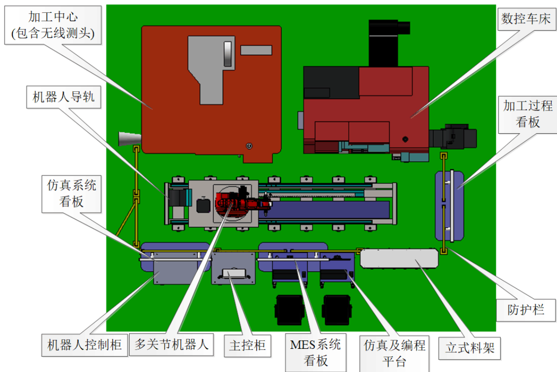
图 2 切削加工智能制造单元技术平台俯视图
