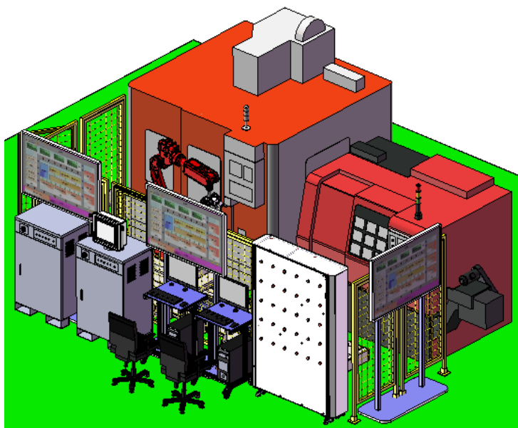
图 1 切削加工智能制造单元技术平台主视图
