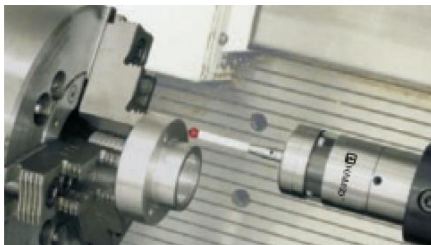
图 6 在线检测示意图
