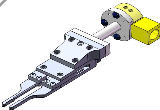
图 9 电极与托盘机器人手爪
