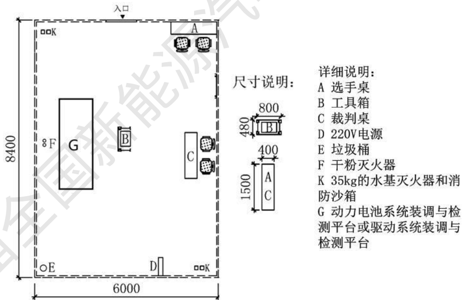
图2 任务1、任务2、任务3和任务5竞赛工位布置图
