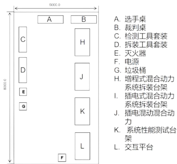
图 1 任务 1、任务 2 竞赛工位布置图
